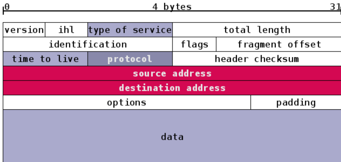
En-tête de paquet IP - image seule 6
