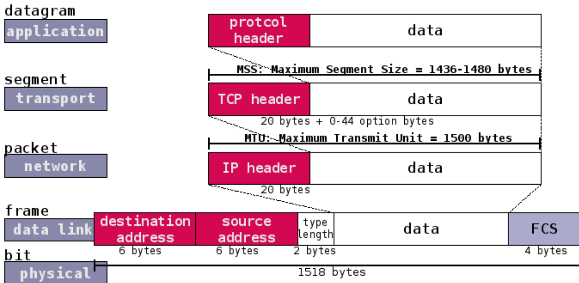
Encapsulation - image seule 5
